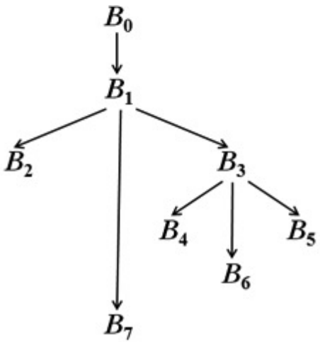
Дерево доминаторов
